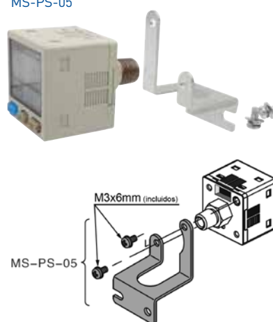
Soporte del sensor MS-PS-05
