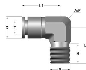
GXLI Codo 90° Tubo-rosca macho BSPT (cónica FIJA)
