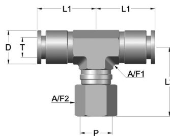
GXTF-G "T" Tubo - Rosca hembra BSPP (cilíndrica orientable) - Tubo
