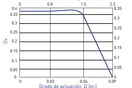
BLQ2 Actuación vs Cv
