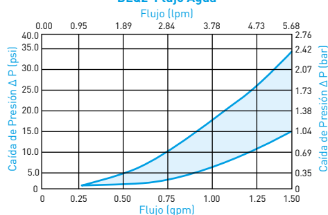
BLQ2 Flujo Agua
