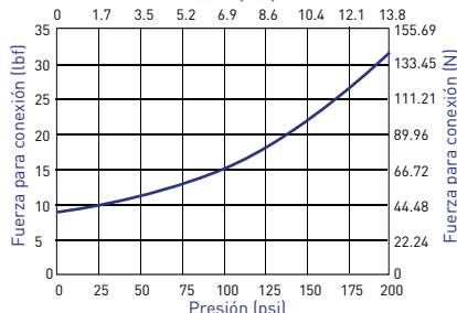
BLQ2 Fuerza para conexión
