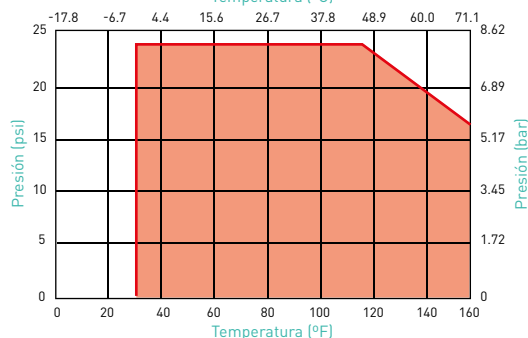
NS4 Rango de Presión Temperatura [°C]
