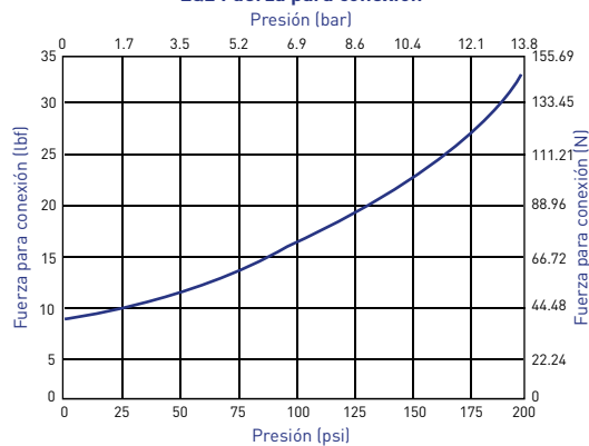
LQ2 Fuerza para conexión
