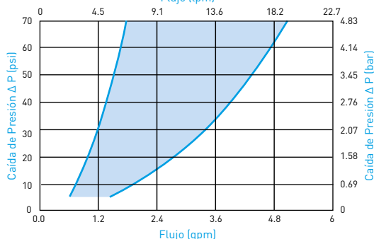
NS4 Flujo Agua Flujo (lpm)
