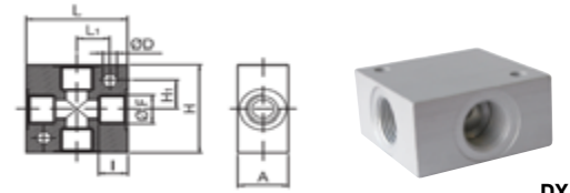
DX Distribuidor cuadrado con salidas en cruz
