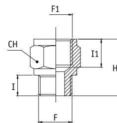
AQI Adaptador Macho cilíndrico BSPP-Hembra cilíndrica BSPP
