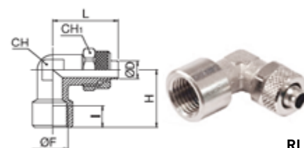
RLF Codo rosca hembra.
