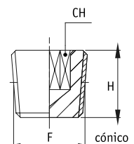
AVB Tapón allen rosca cónica BSPT enrasado
