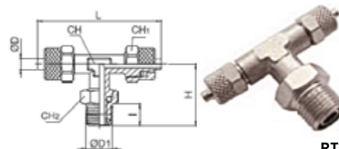
RTR "T" Central giratoria rosca cónica.
