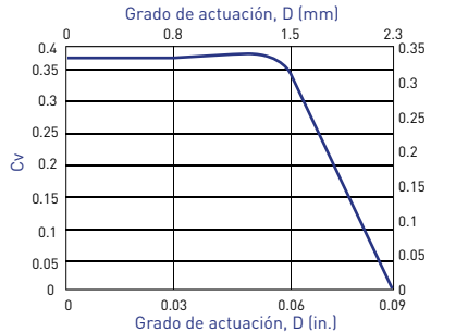
BLQ2 Actuación vs Cv
