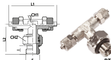
RTG "T" Central giratoria rosca cilíndrica con junta.
