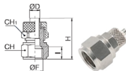
RCF Rosca hembra.
