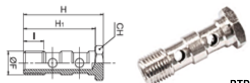
RTD Tornillo doble.
