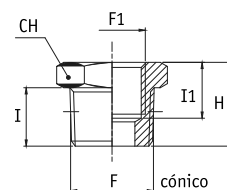
AR Reducción Rosca Macho BSPT-Hembra cilíndrica BSPP
