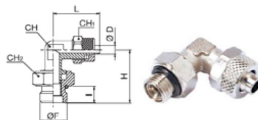
RLG Codo macho cilíndrico giratorio, con junta tórica.
