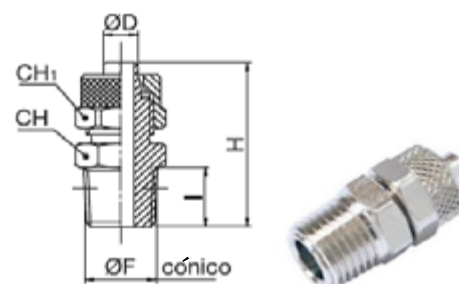
RC Macho cónico.
