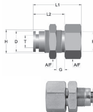
GXMF-G Recto Tubo-Rosca hembra pasamuros BSPP (cilíndrica)
