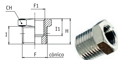
AR Reducción Rosca Macho BSPT-Hembra cilíndrica BSPP
