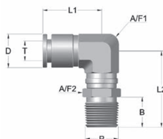
GXL Codo 90° Tubo-rosca macho BSPT (cónica orientable)
