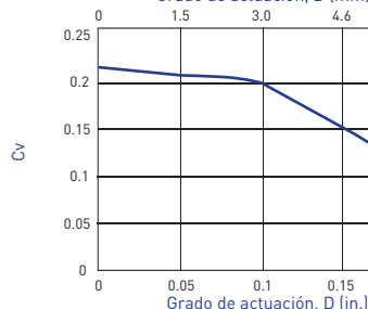
BLQ6 Actuación vs Cv
