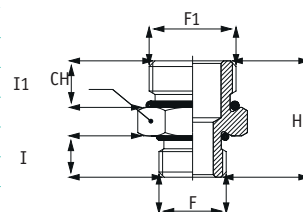
ACJ Machón rosca cilíndrica BSPP junta NBR
