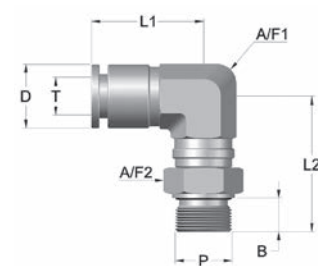
GXL-G Codo 90° Tubo-rosca macho BSPP (cilíndrica orientable)
