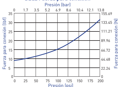
BLQ2 Fuerza para conexión
