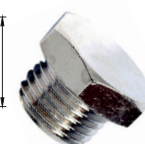
AV Tapón hexagonal hueco Macho cilíndrico BSPP sin junta
