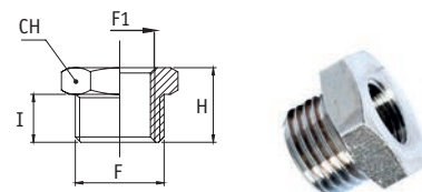
ARI Reducción Rosca Macho-Hembra cilíndrica BSPP
