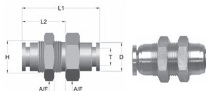
GXMM Unión Tubo-Tubo pasamuros.
