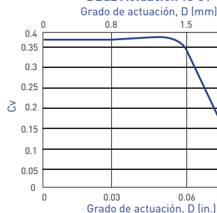
BLQ2 Actuación vs Cv
