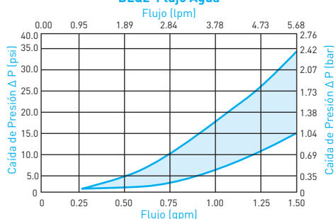
BLQ2 Flujo Agua
