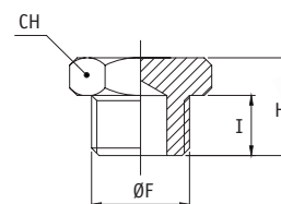
AV Tapón hexagonal hueco Macho cilíndrico BSPP sin junta
