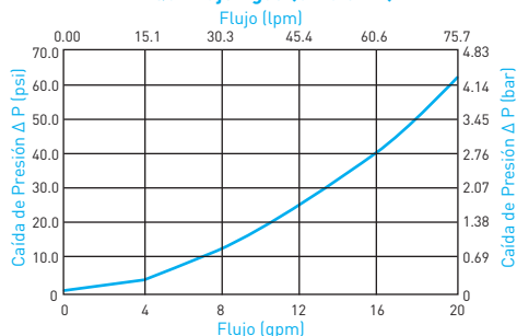
BLQ6 Flujo Agua (0-20 GPM)
