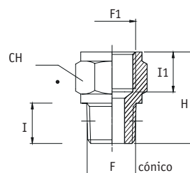
AQ Adaptador Macho cónico BSPT-Hembra cilíndrica BSPP
