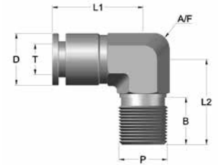
GXLI Codo 90° Tubo-rosca macho BSPT (cónica FIJA)
