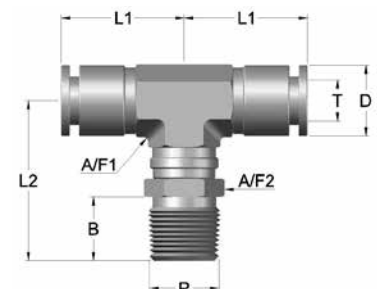
GXT "T" Tubo - Rosca macho BSPT (cónica orientable) - Tubo
