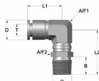
GXL Codo 90° Tubo-rosca macho BSPT (cónica orientable)
