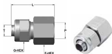
RCFX Recto rosca hembra cilíndrica BSPP
