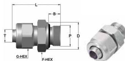
RCIX -G Recto rosca macho cilíndrica BSPP
