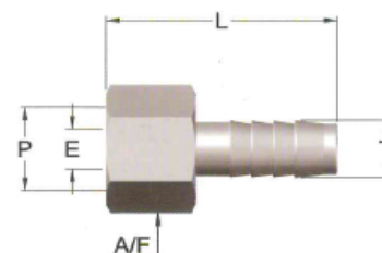
AXEBP Rosca hembra cilíndrica BSPP
