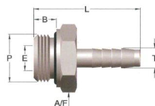
AXEACP-G Rosca macho cilíndrico BSPP-VITÓN
