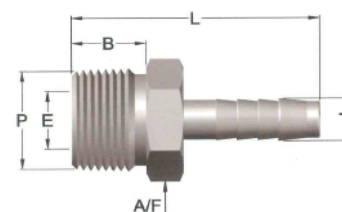
AXEACP Rosca macho cónico BSPT
